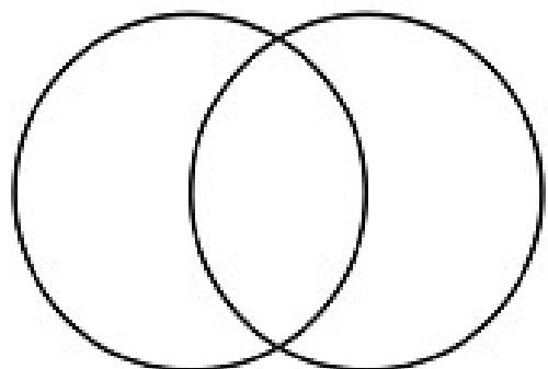
VENN DIAGRAM
